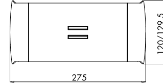
L. 275 P. 120 H. 73
